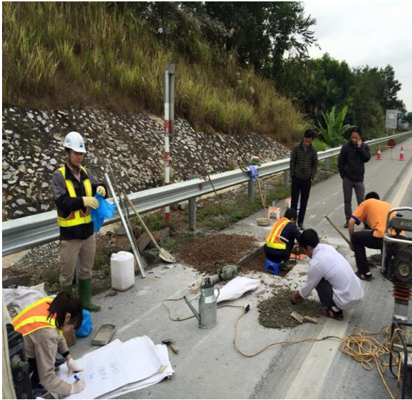
Thí nghiệm kiểm định dự án đường cao tốc Nội Bài - Lào Cai (Phục vụ Hội đồng nghiệm thu Nhà nước)
